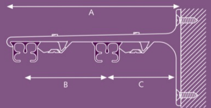
Wall bracket aluminium double A) 15 cm (6''), B) 9,2 cm (3,6''), C) 4,5 cm (1,8'') A) 20 cm (8''), B) 9,2 cm (3,6''), C) 9,5 cm (3,7'')
